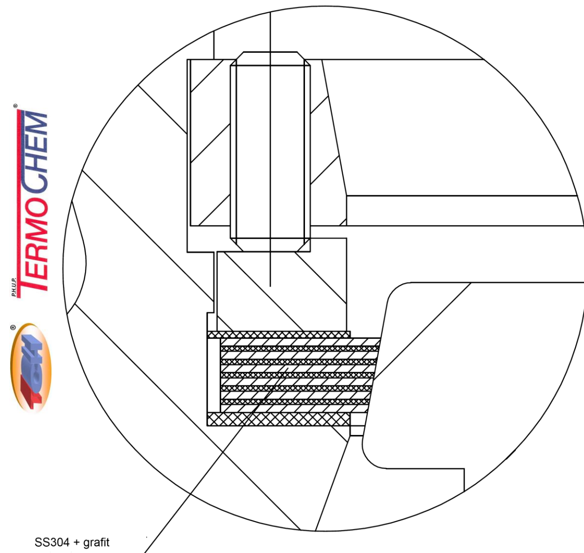
uszczelnienie lamelowe
