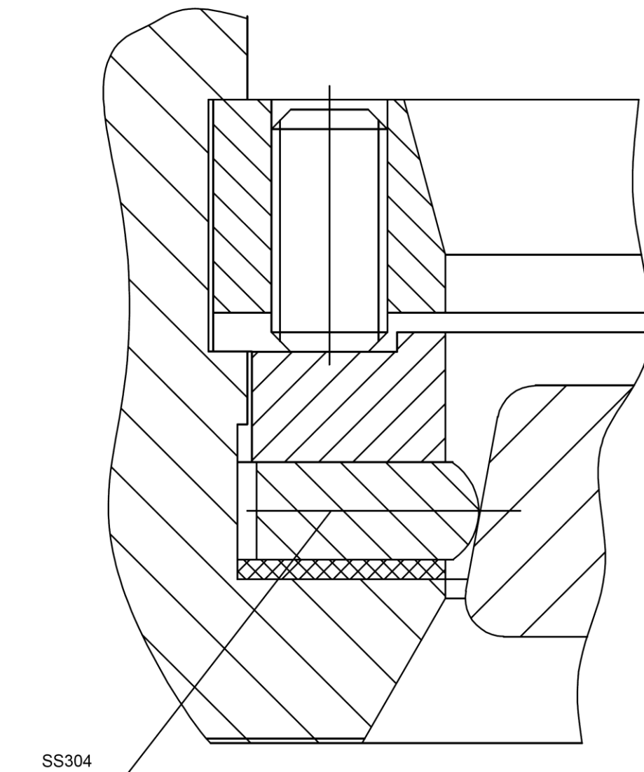
uszczelnienie metal/metal (pierścień SS304)
