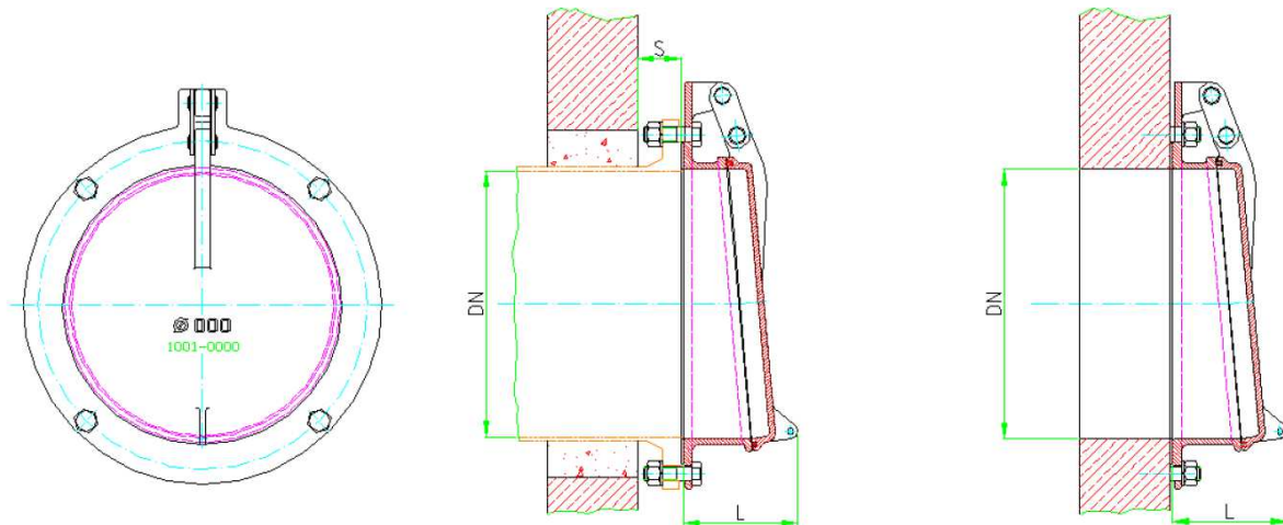
Wersja kołnierzowa (do kołnierza DIN 2501 PN10)
